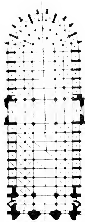
Plan de Notre-Dame de Paris.
